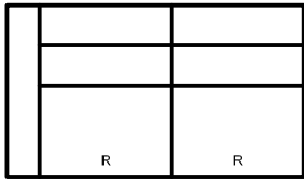
Terminale 3 Posti (SX/DX) L 180 x P 104 x A 81/103 (sedute 80cm)
