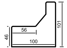
Haut. assise : 46 cm Prof. assise : 56 cm Haut. accoudoir : 67 cm
