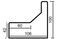
Haut. assise : 42 cm Prof. assise : 60 cm
