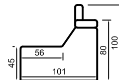
Alt. di seduta : 45 cm Prof. di seduta : 56 cm
